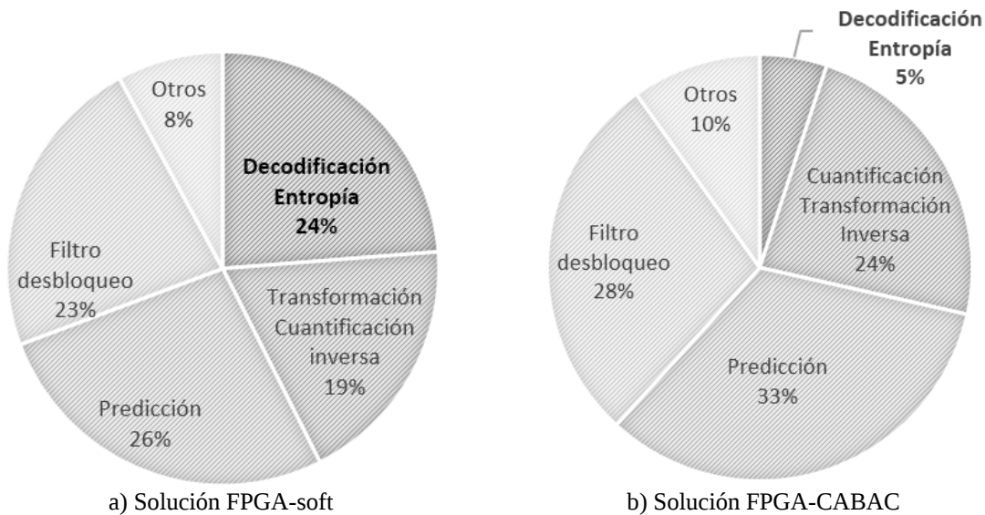
Figura 6: Porcentaje de tiempo de procesamiento de los bloques del Decodificador H.264/AVC para el video 4.c
