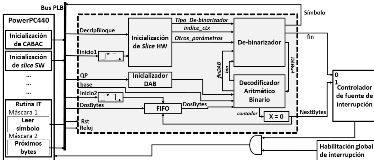
Figura 3: Diagrama en bloques del diseño del módulo IP Decodificador CABAC y su interacción con el procesador
