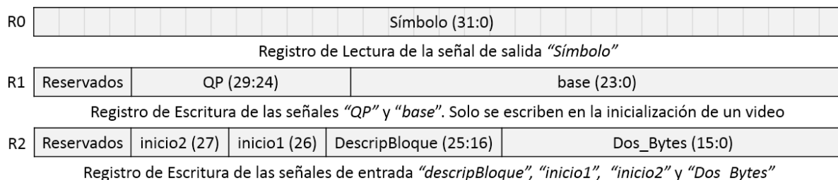
Figura 5: Registros de Lectura/Escritura para la comunicación con el módulo IP diseñado
