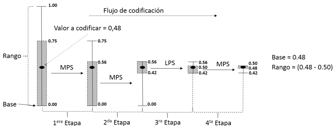
Figura 1: Ejemplo de un proceso de codificación de entropía por el método definido por CABAC
