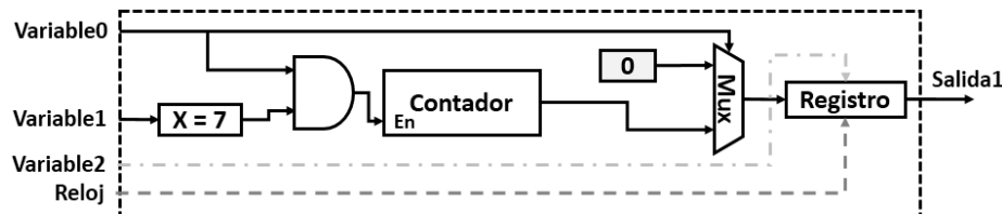
Figura 4: Planteamiento del diseño de cada señal de salida en los bloques propuestos en el módulo IP Decodificador CABAC
