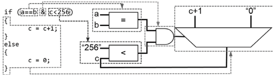
Figura 2: Metodología de interpretación a VHDL de instrucciones en lenguaje C
