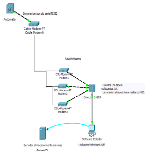
Fig.3 Diagrama de dispositivos del nuevo sistema OpenSiger.
